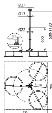
Maßbild V DBS RA320 PAE 27 V 600 1180
