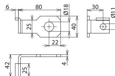
Maßbild AB EXFS IF1 W 18
