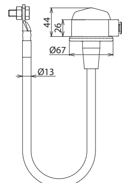
Maßbild EXFS L300
