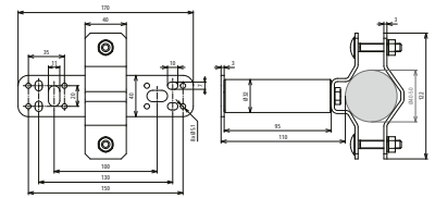
Maßbild WB D40.50 SE WA110 V2A
