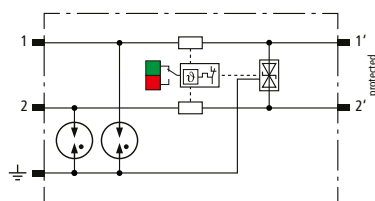
Prinzipschaltbild BCO MOD ML2 BE HF 24
