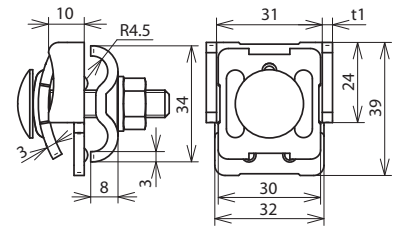
Maßbild FK DUL 8.10 KBF0.7 8 CU
