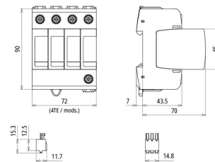
Maßbild DG MD TNS ACI 275 FM
