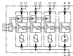
Prinzipschaltbild DG MD TNS ACI 275 FM
