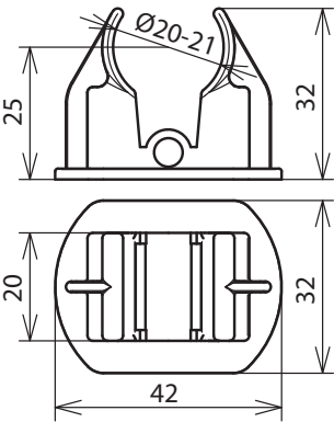
Maßbild RLA 20 FB K SW
