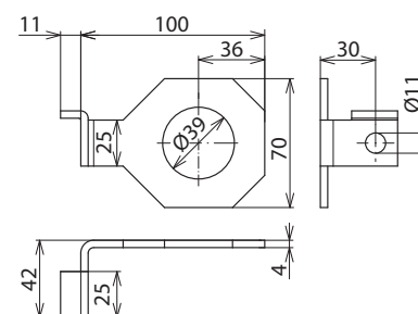
Maßbild AB EXFS IF1 W 39
