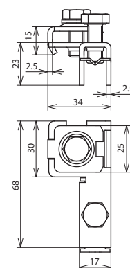
Maßbild SPK 25 BRS AK1X10 2X6.8 V2A
