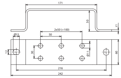
Maßbild ES 2X3 ASB11 STTZN
