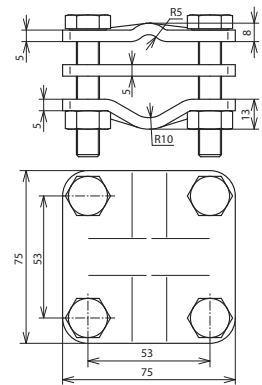
Maßbild AK TE 20.30 8.12 FL40 STTZN
