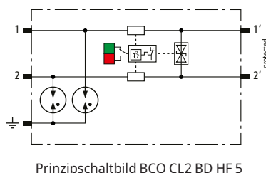
Prinzipschaltbild BCO CL2 BD HF 5
