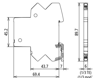
Maßbild BCO CL2 BD HF 5
