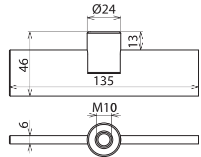
Maßbild KM AB M10 SN7280
