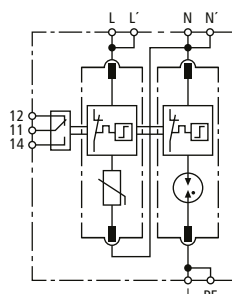
Prinzipialschaltbild DG MP TT 2P 275 FM
