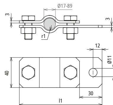
Maßbild ERS 55 AB11 STTZN
