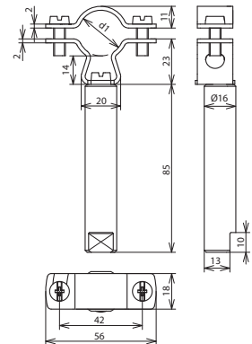
Maßbild LH ZS 20 23 KT D16 L85 V2A
