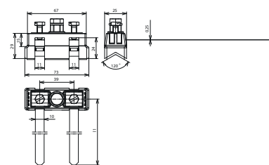
Maßbild EX BRS 27
