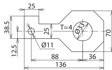
Maßbild AB EXFS IF3 G 33
