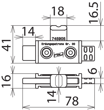
Maßbild EP NH00 VI TA
