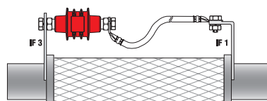
Prinzipschaltbild EXFS 100
