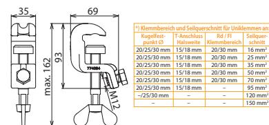
Maßbild UEK 25 FS
