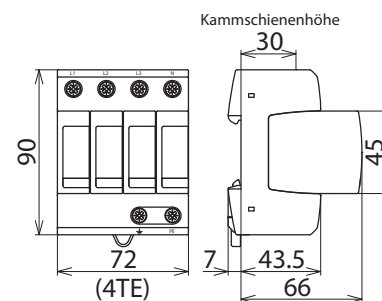
Maßbild DG M H TT 275
