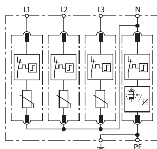
Prinzipschaltbild DG M H TT 275
