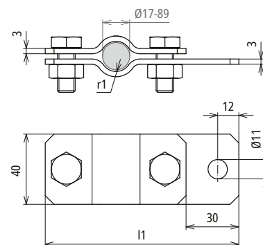
Maßbild ERS 17 AB11 STTZN
