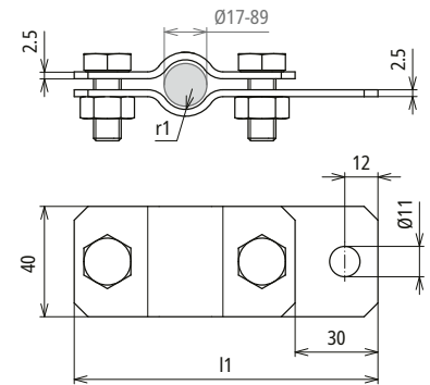
Maßbild ERS 89 AB11 V2A
