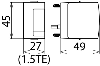
Maßbild DG MOD E DC 60
