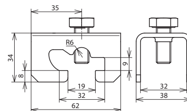
Maßbild VK EH R10 F30 V2A
