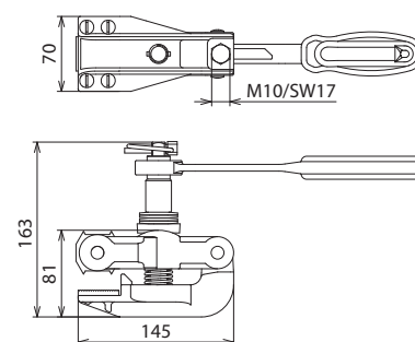
Maßbild SAK PFE ARA
