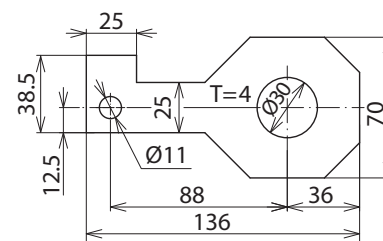
Maßbild AB EXFS IF3 G 30
