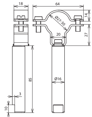
Maßbild LH ZS 27 KT D16 L85 V2A
