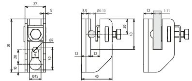
Maßbild FRH 11 6.10 WA15 B7 STTZN
