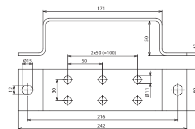
Maßbild ES 2X3 ASB11 V2A
