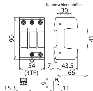
Maßbild DG M WE 600 FM
