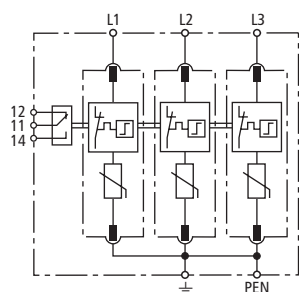
Prinzipschaltbild DG M WE 600 FM
