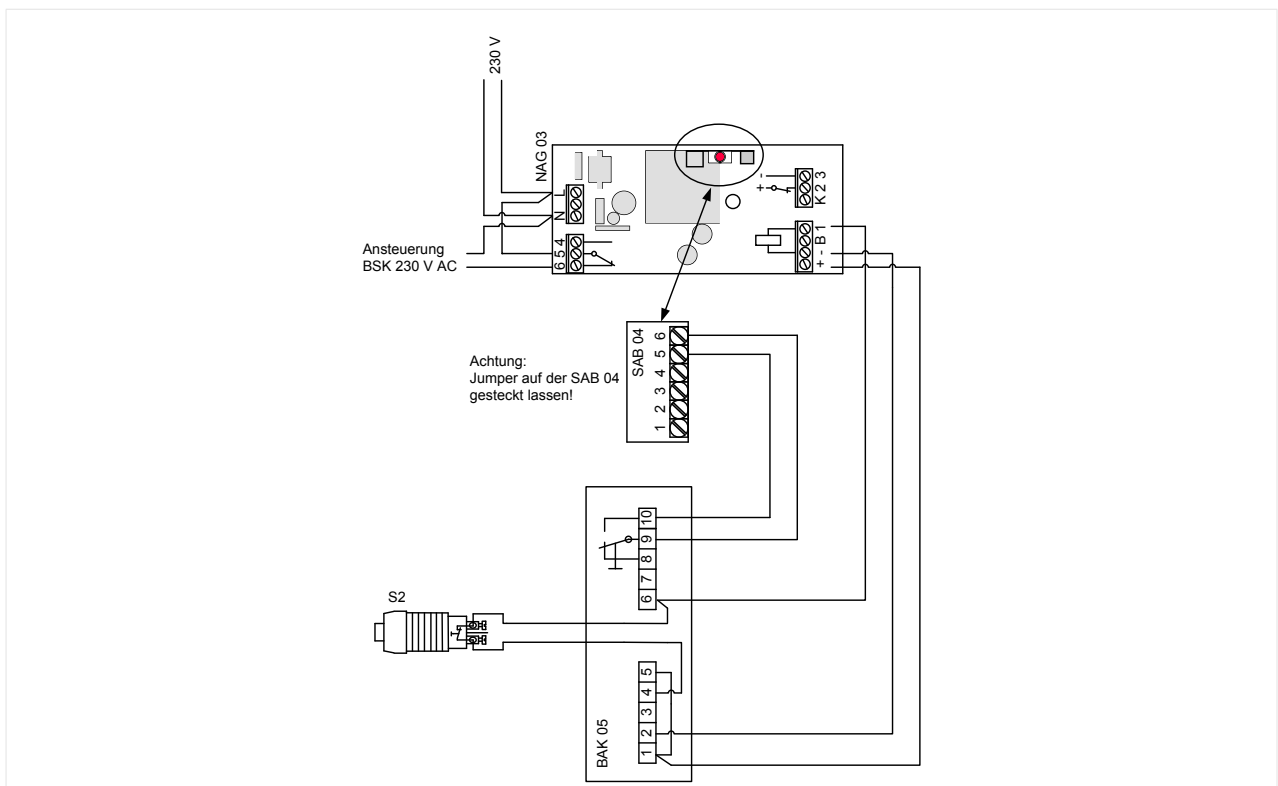
Abb. 8: Ansteuerung des LRS 03 über ein NAG 03 mit SAB 04
