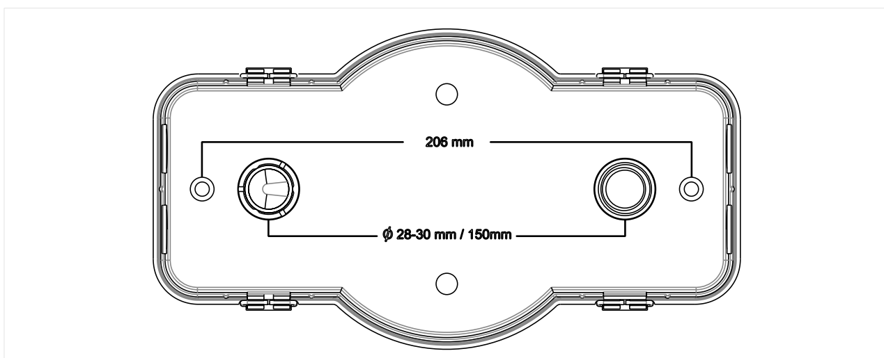
Abb. 5: Bohrmaße
