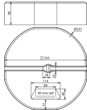
Maßbild BES 17KG KT16 D337
