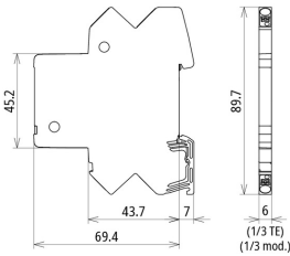
Maßbild BCO CL2 BE HF 5
