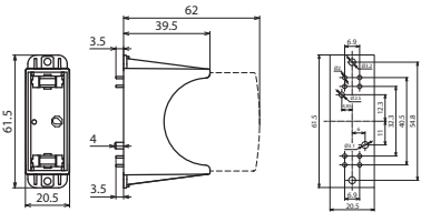
Maßbild DG PCB PV SCI 500
