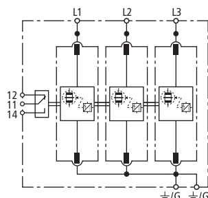
Prinzip Schaltbild DB MU 3PY 208 3W+G R
