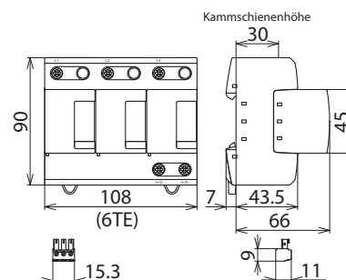
Maßbild DB MU 3PY 208 3W+G R
