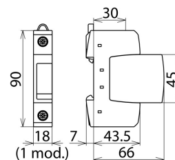
Maßbild DG SU 1P 120
