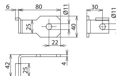
Maßbild AB EXFS IF1 W 11
