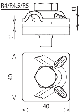
Maßbild MVK 10 SKM10X35 STTZN
