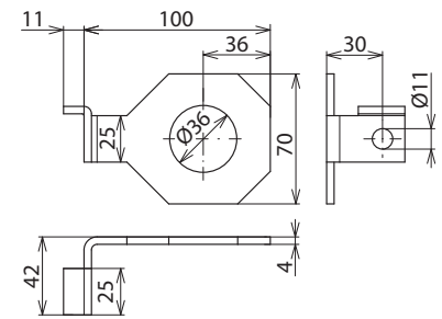
Maßbild AB EXFS IF1 W 36
