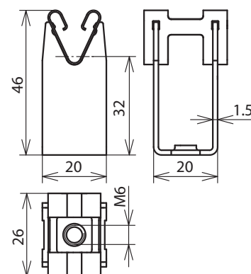
Maßbild LH DG 8 H32 IGM6 CU
