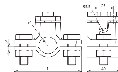
Maßbild ERS 60 AS4.10 TG STTZN
