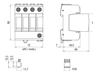
Maßbild DG MD TT 150 FM
