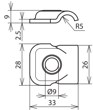
Maßbild KB 6.10 B9 STTZN
