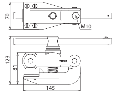
Maßbild SAK PFE KN AB29
