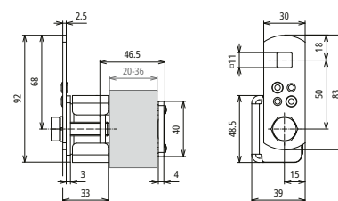
Maßbild AKK AL B11.11 KBF 20 36 STTZN
