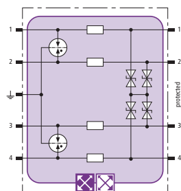
Prinzipschaltbild BXT ML4 BC 5
