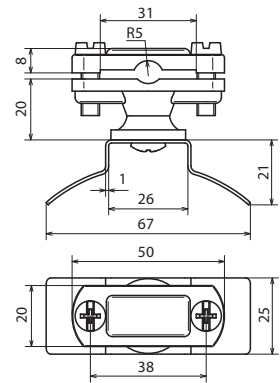
Maßbild LH ZS 6.11 FL30 SBB PA V2A
